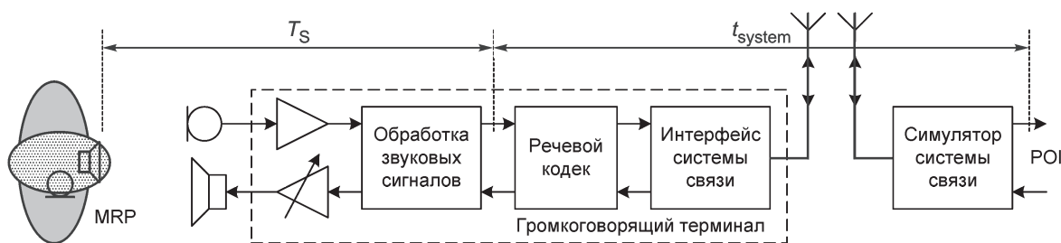
Рисунок 6 — Задержка распространения сигнала в канале передачи
