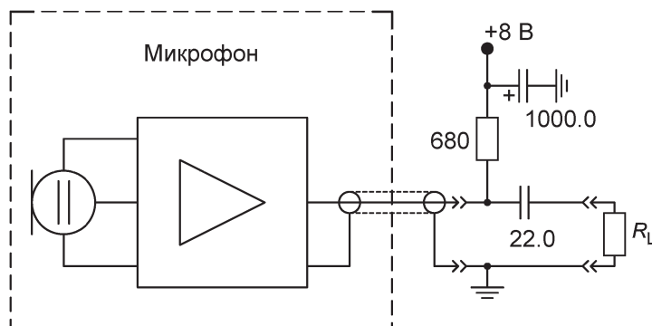
Рисунок 2 — Блок-схема испытательной установки для микрофонов
