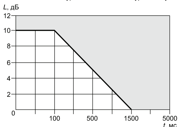
Рисунок 9 — Зависимость отношения остаточного уровня эхо-сигналов к уровню шума паузы от времени
