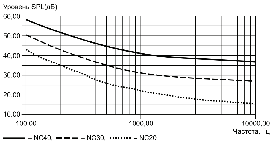
Рисунок 4 — Спектральная плотность окружающего шума
