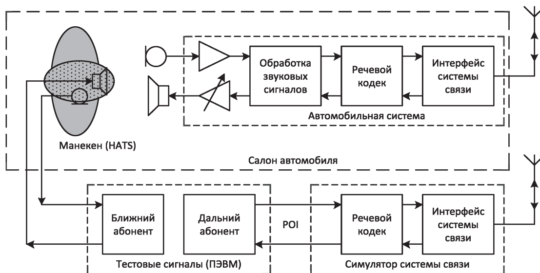
Рисунок 1 — Блок-схема установки для испытания автомобильной системы
