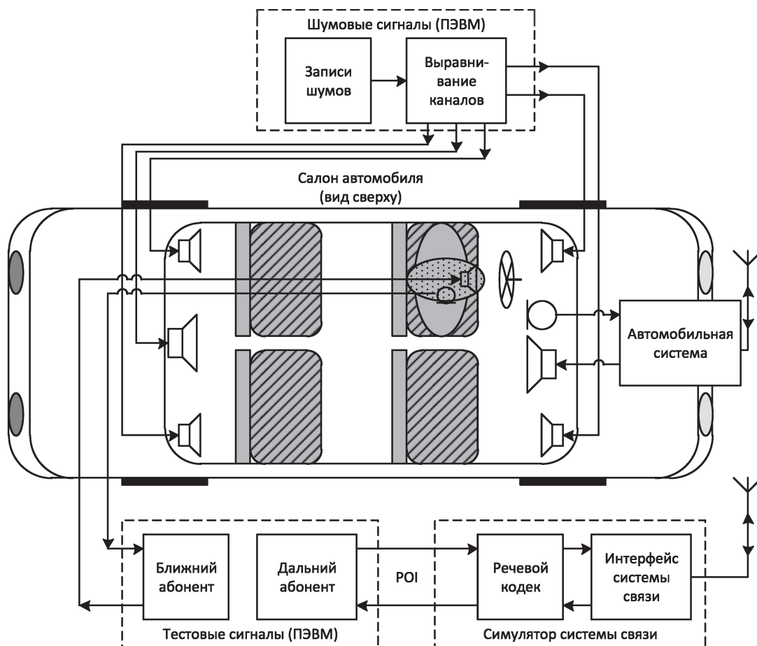
Рисунок 3 — Тестовое оборудование для имитации внешнего акустического шума
