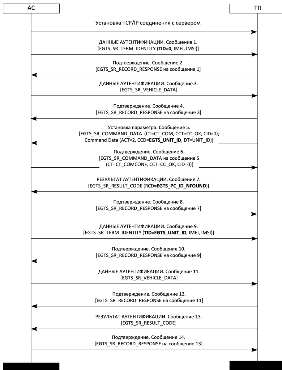
Рисунок 9 — Алгоритм конфигурации УСВ с использованием GPRS
