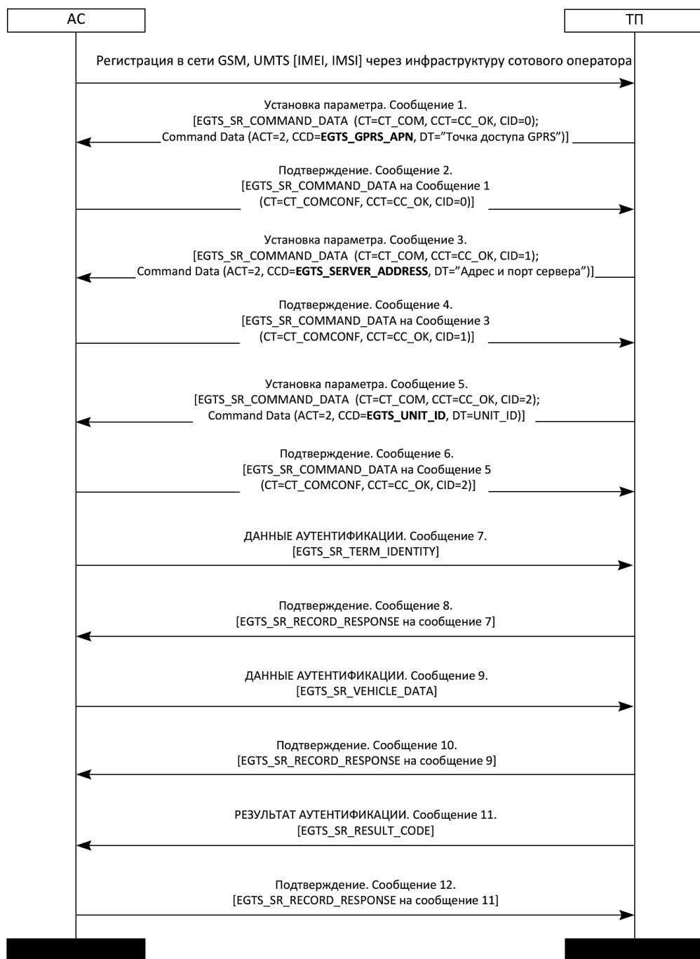
Рисунок 8 — Алгоритм конфигурации УСВ с использованием SMS
