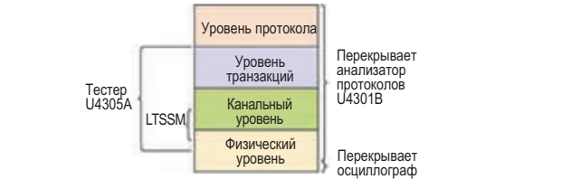
Уровни сетевой модели OSI, перекрываемые модулем тестера PCIe 3.0 U4305A
