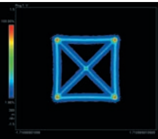
I/Q-диаграмма
