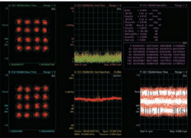
Y-поляризация: диаграмма созвездия сигнала с модуляцией 16-QAM Х-поляризация: спектр вектора ошибки Х-поляризация: уровни амплитуды сигнала
