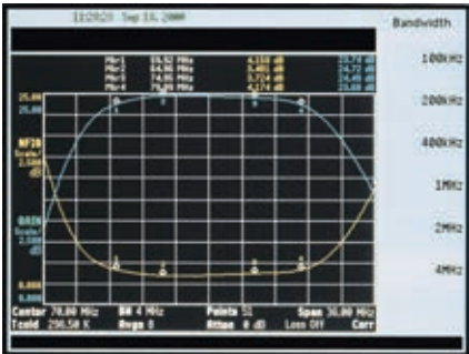
Встроенный цветной дисплей с диагональю 17 см обеспечивает одно- или полиэкранное отображение результатов одновременного измерения коэффициента усиления и коэффициента шума.
