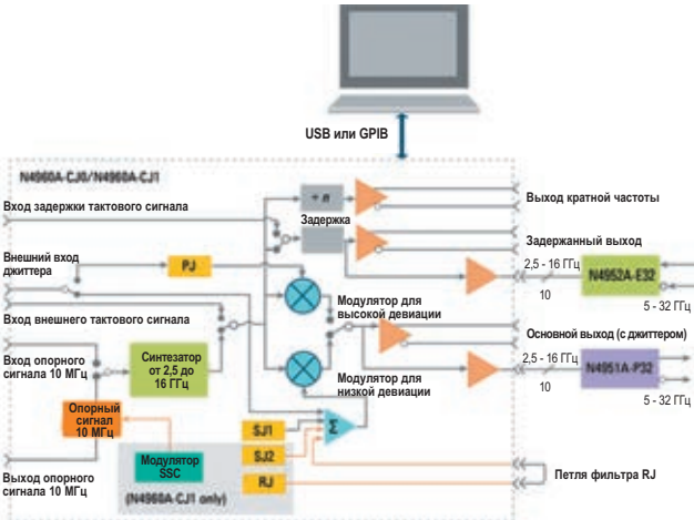
Структурная схема системы тестирования до 32 Гбит/с
