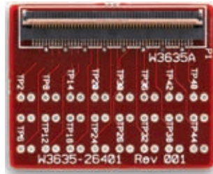
Плата-адаптер осциллографических пробников W3635A с контрольными точками для подключения к осциллографу
